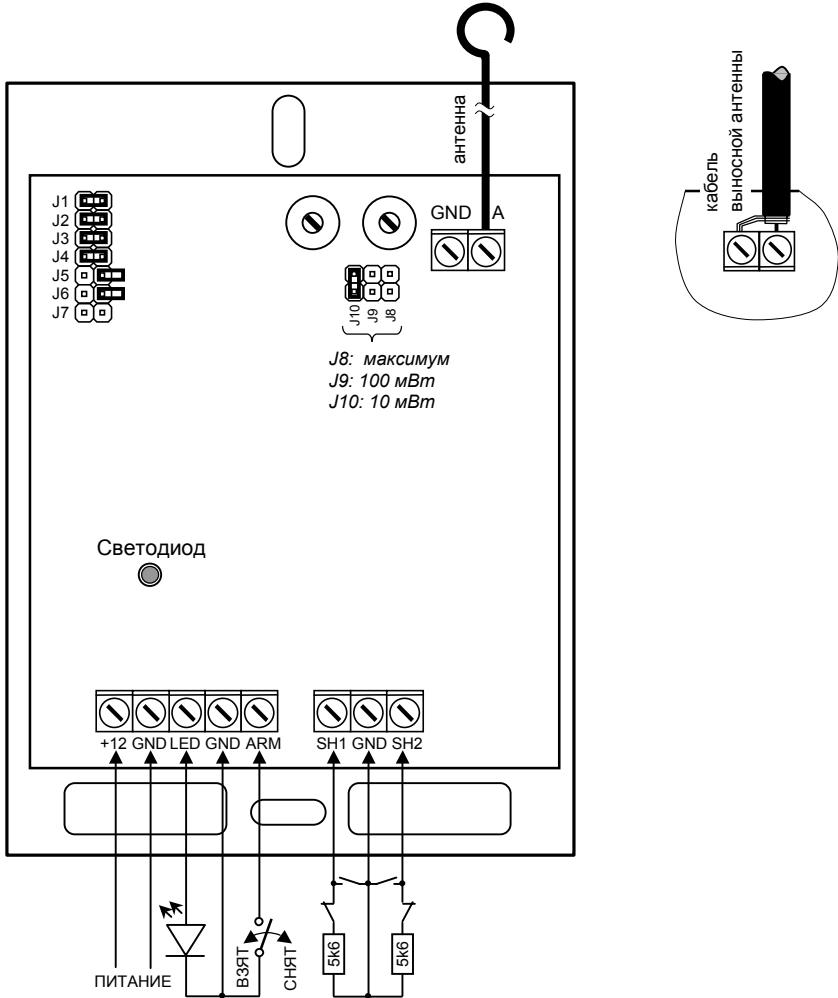
Рис. 2. Монтажная схема передатчика и подключение антенны
